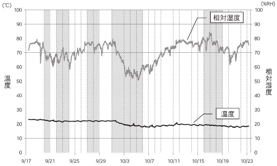
図9 1階南側廊東端の小室 (H15) の温度湿度の変動
