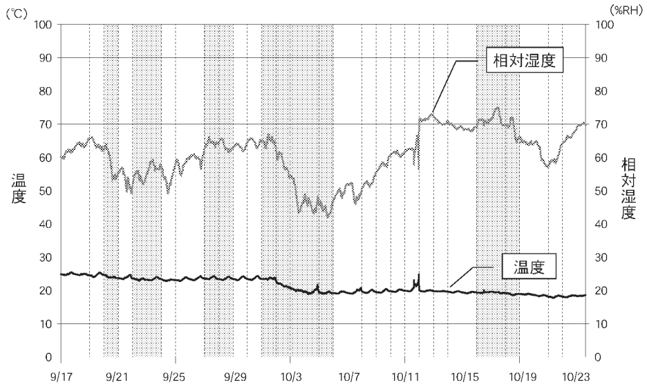
図11 2階北側廊 (H 8) の温度湿度の変動
