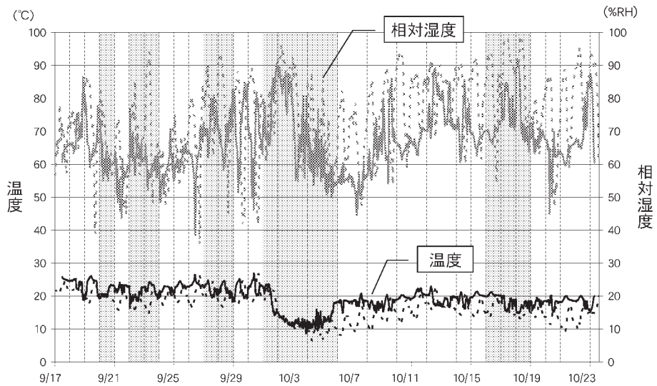
図12 2階西側廊南窓 (H13) と堂外の温度湿度の変動比較 (点線が堂外 (OutH) の温度湿度)
