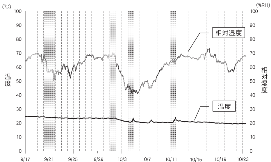
図20 コンサート開催日のアプシスH 4 の温度湿度の変動
