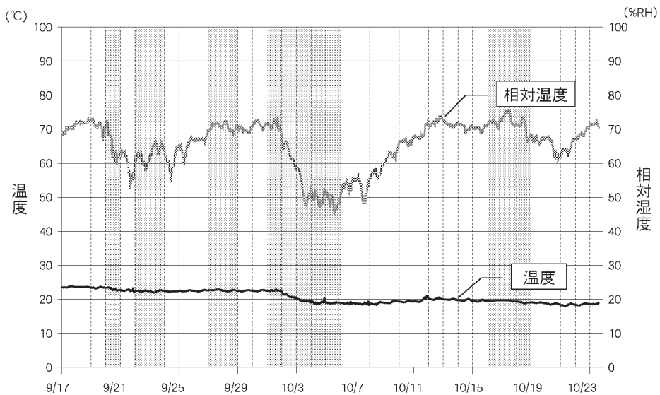
図8 1階ナルテクス (H 3) の温度湿度の変動
