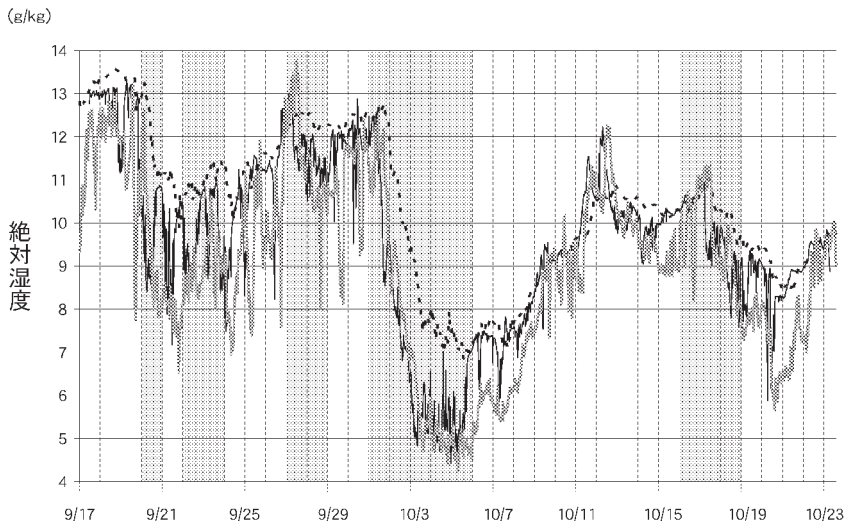
図14 1階身廊南ピア (H6) と2階西側廊南窓 (H13)、外気 (OutH) の絶対湿度の変動比較 (黒点線: H6 (1階身廊南ピア), 黒太線: H13 (2階西側廊南窓), 灰色: OutH (外気))
