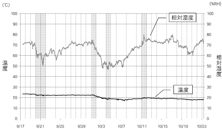
図19 コンサート開催日の入口H 9 の温度湿度の変動
