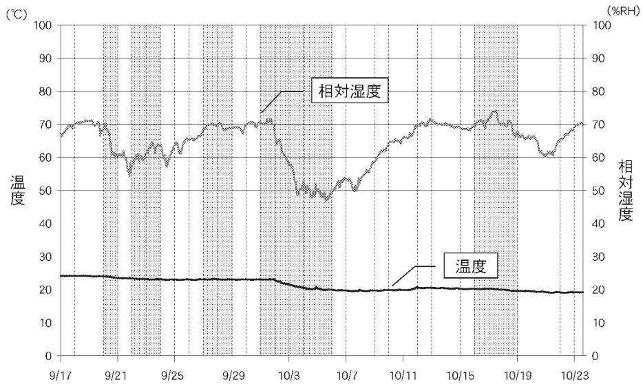
図7 1階身廊南ピア (H 6) の温度湿度の変動
