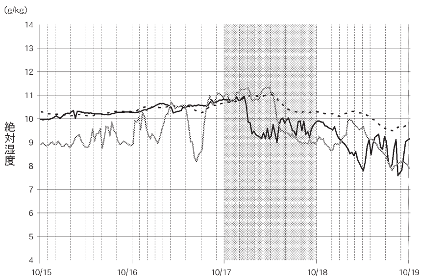
図16 10月17日の1階身廊南ピア (H 6) と2階西側廊南窓 (H13), 外気 (OutH) の絶対湿度の変動比較 (黒点線: H 6 (1階身廊南ピア), 黒太線: H13 (2階西側廊南窓), 灰色: OutH (外気))
