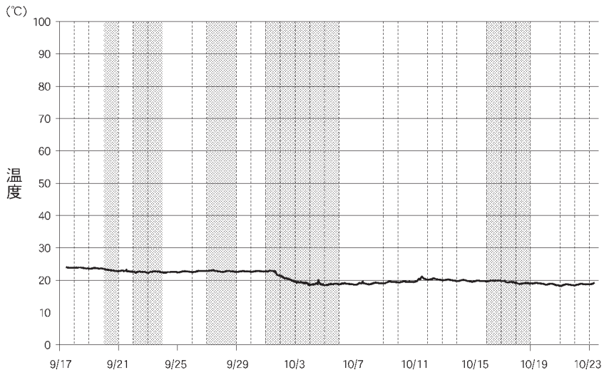
図13 2階階段上 (H10) の温度の変動
