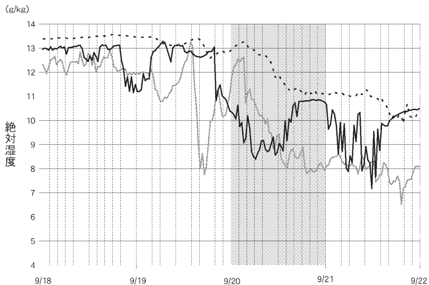
図15 9月20日の1階身廊南ピア (H 6) と2階西側廊南窓 (H13), 外気 (OutH) の絶対湿度の変動比較 (黒点線: H 6 (1階身廊南ピア), 黒太線: H13 (2階西側廊南窓), 灰色: OutH (外気))
