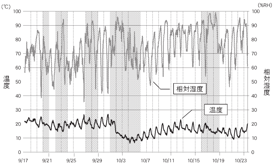
図6 堂外（アトリウム・中庭（OutH））の温度湿度
