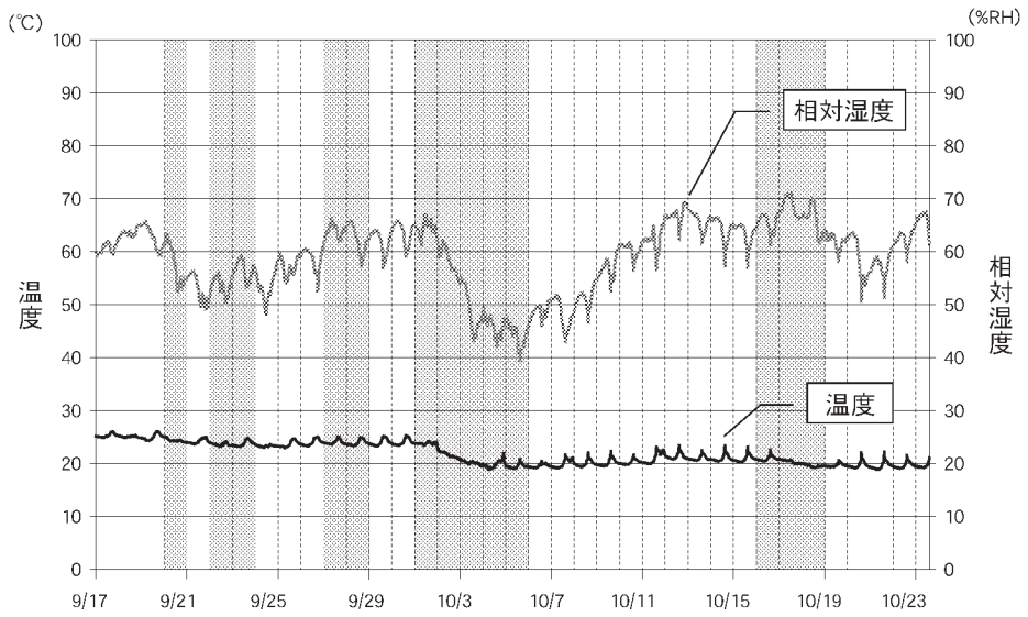
図10 2階南側廊 (H7) の温度湿度の変動
