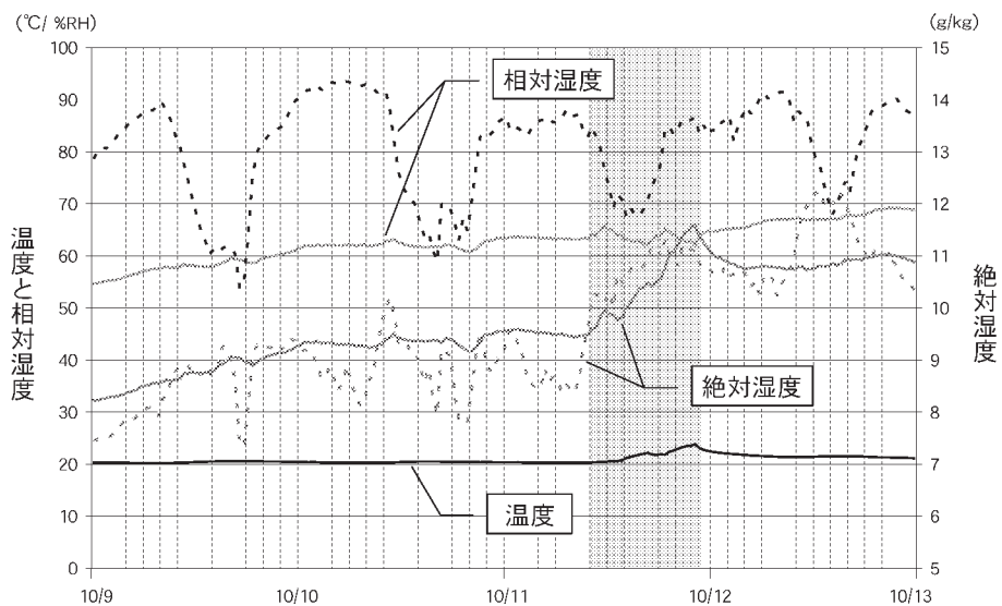
図22 10月11日のアプシスH 4と外気 (OutH) の温度、相対湿度ならびに絶対湿度の変動 (実線：H 4 (アプシス), 点線：OutH (外気))
