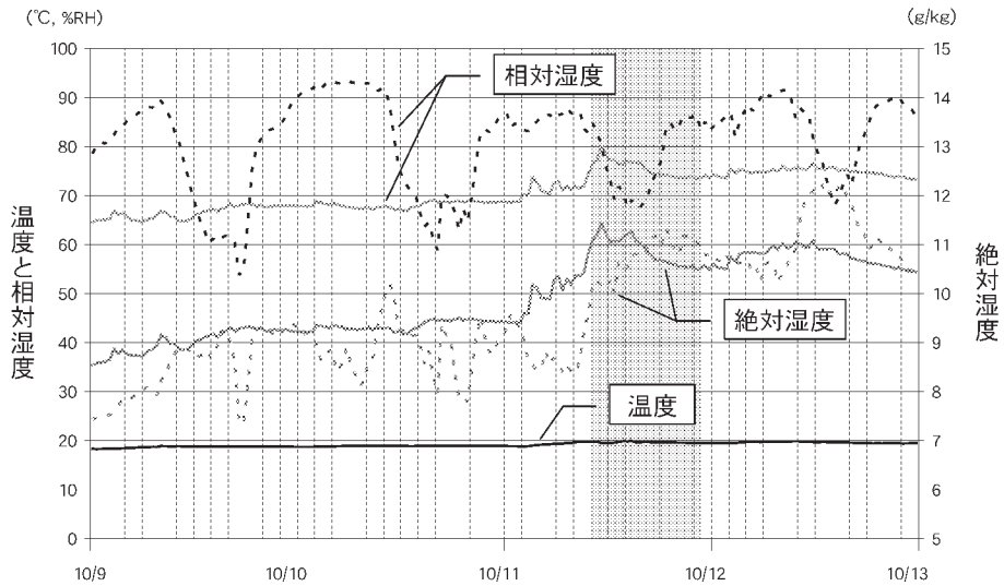
図21 10月11日の入口H 9と外気 (OutH) の温度、相対湿度ならびに絶対湿度の変動比較 (実線：H 9 (入口), 点線：OutH (外気))
