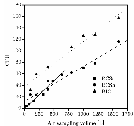
図1 サンプリング吸引量と捕集真菌数
