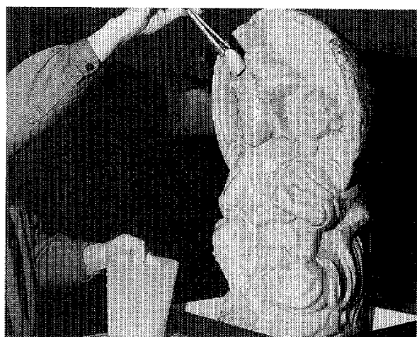
写真-6 撥水性シランの塗布含浸処置
