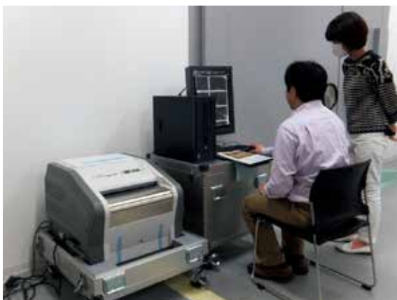
可搬型現像装置を用いたX線透過撮影調査 （サントリー美術館）
