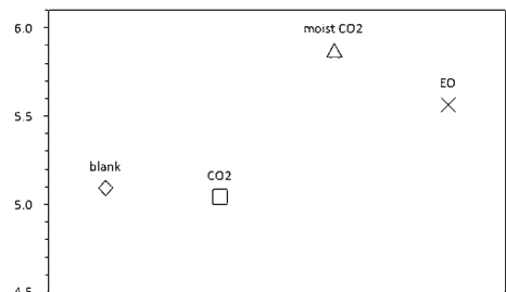
図 8 ガス処理によるシアノタイプの pH の変化
