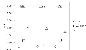
図4 ガス処理がジアゾタイプの色(blankとの色差ΔE)に及ぼす影響
