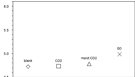
図 7 ガス処理によるジアゾタイプの pH の変化
