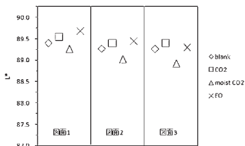
図1 ガス処理がジアゾタイプの試料の色(L値)に及ぼす影響
