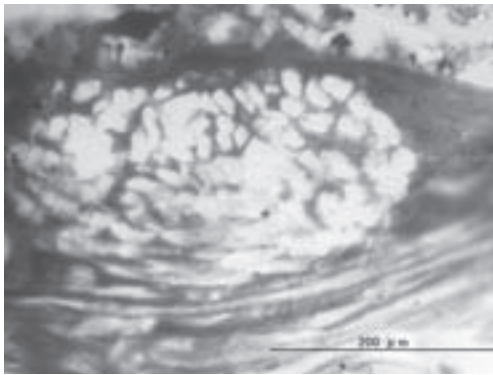
図9 下地部分にみられる布着せ補強の繊維断面（1）
