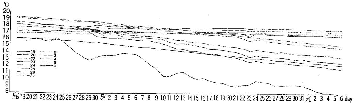
図-11 土中、石室の温度変化（昭和57年11月18日～昭和58年1月5日）
