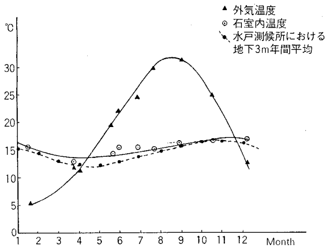
図一 2 未開口石室内の温度曲線（昭和48年～昭和55年）
