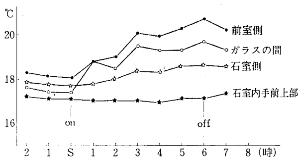
図一 9 二重ガラスによる断熱効果
