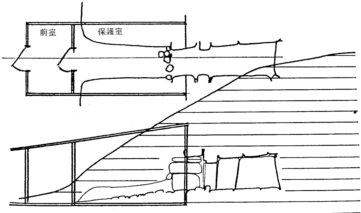
図一 3 仮設保護室図
