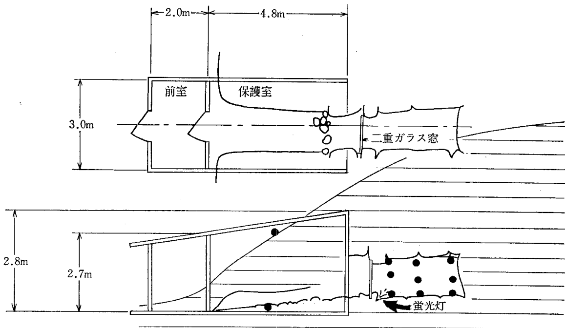
図一 仮設保護室平面図
