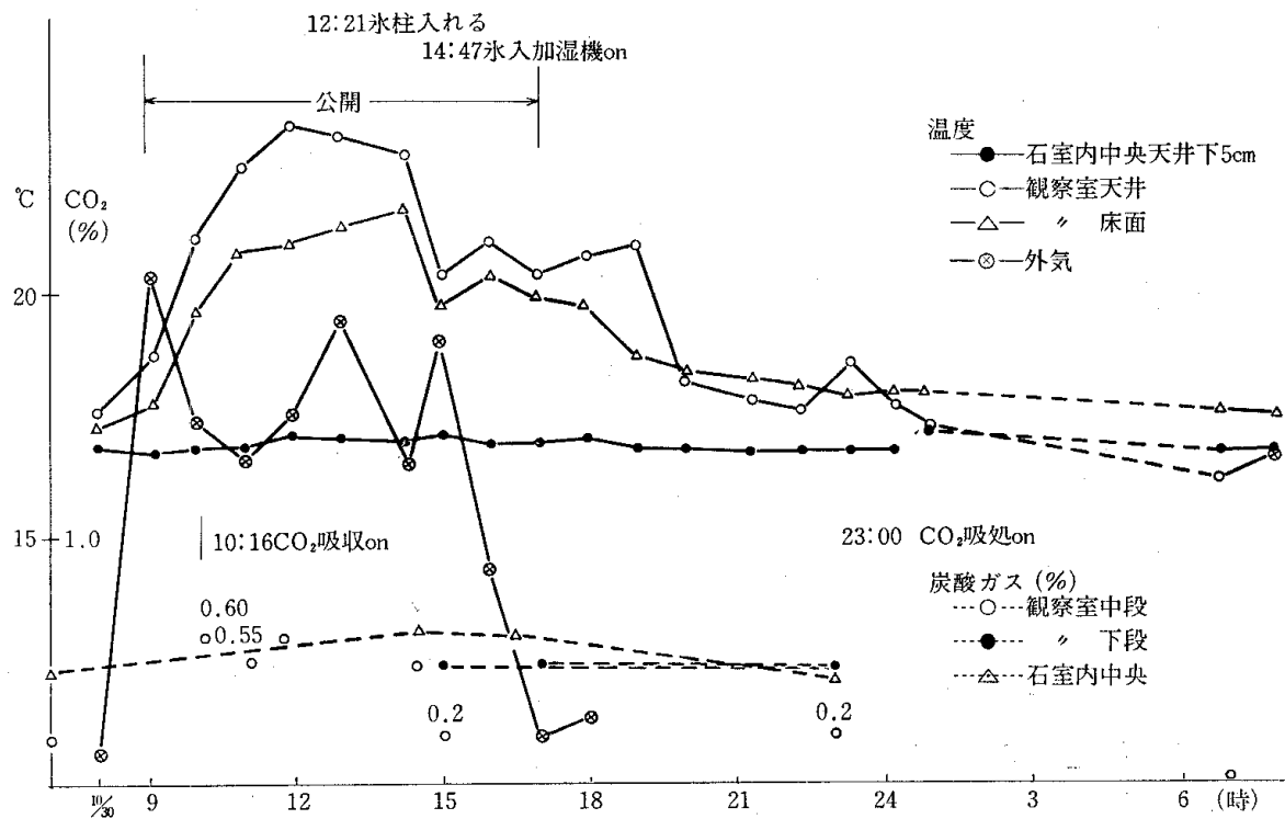
図一八 一般公開時の環境測定結果
