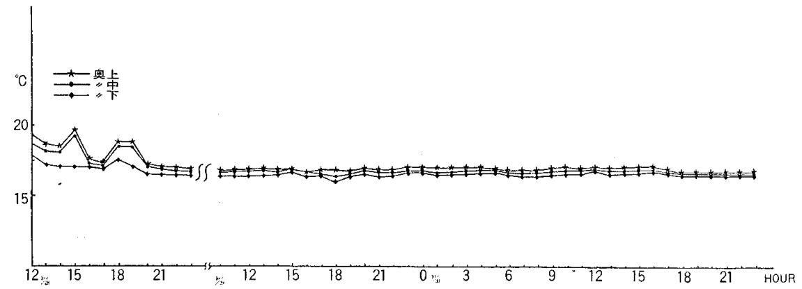
図一6 石室内（奥）温度曲線（仮施設）
