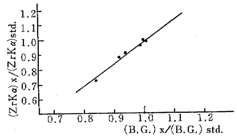
図3 ZrK_{\alpha} ピーク高とバックグラウンドに対するマトリックス効果
