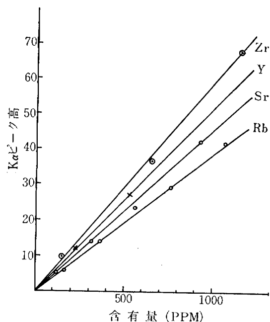
図-2 ルビジウム，ストロンチウム，イットリウム，ジルコニウムの検量線
