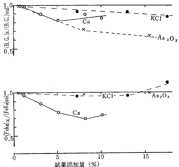
図4 FeK_{\alpha} およびバックグラウンドに対するマトリックス効果
