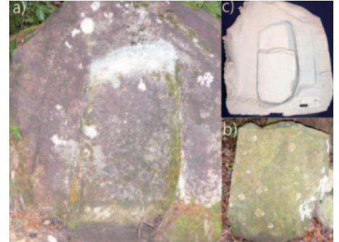
今は離れた場所にある枠石(a)と石碑残欠(b)とを三次元計測し、過去に行われた石碑の修復行為を模型によって検証しました(c)
